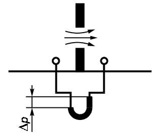
Рисунок А.7 — Принцип перепада давления
