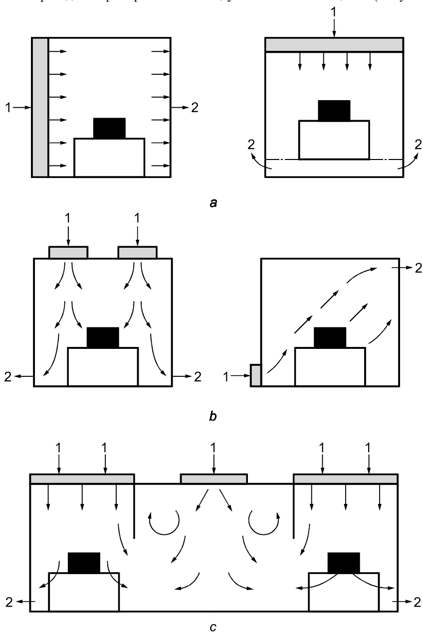
а — однонаправленный поток воздуха; б — неоднаправленный поток воздуха; в — смешанный поток воздуха; 1 — приточный воздух; 2 — вытяжной воздух
